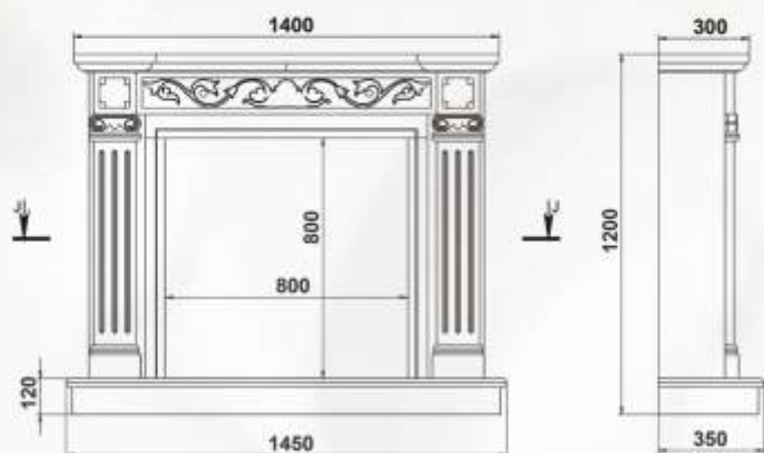
J-J (1 : 12)
