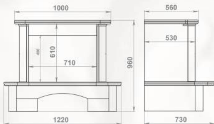
чертеж облицовки под топку 700-й серии
